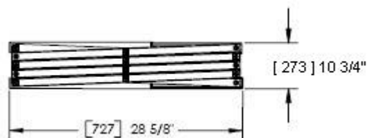
Vue latérale / hauteur minimale, sans montage
