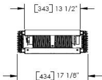
Vue avant/largeur
