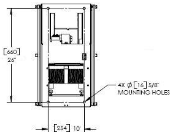
Vue de dessus/modèle de
