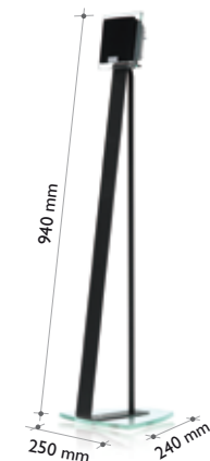
Sério sur pieds (option) 3 couleurs au choix (noir, gris, blanc)
