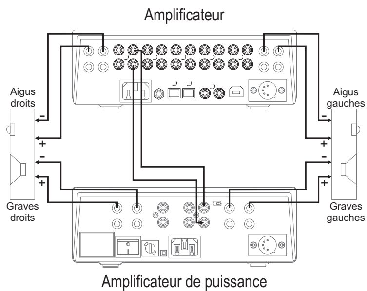
Raccordement d'un système d'enceintes bi amplifié
