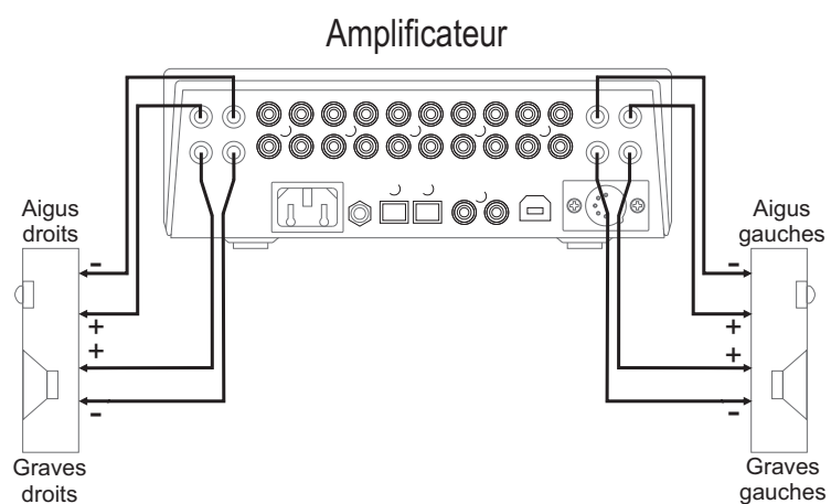
Raccordement d'un système d'enceintes bi câblé
